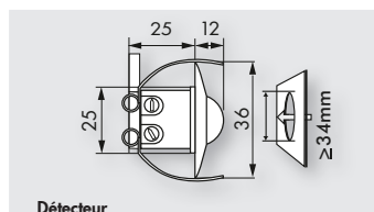
Détecteur
